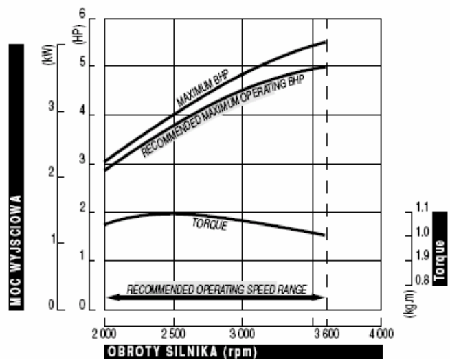
Wykres osiągow
